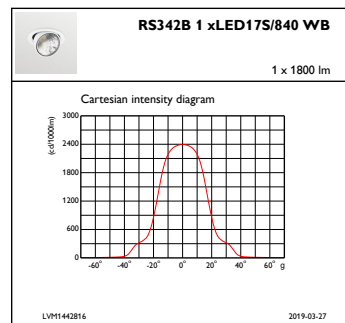
IFCC1_RS342B1xLED17S840WB
